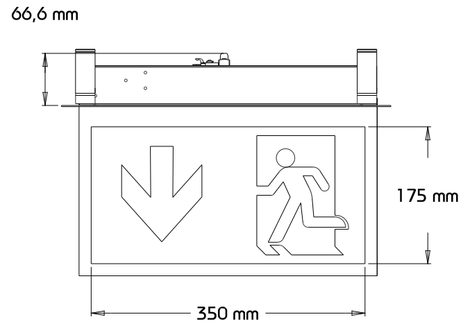
Ansicht Hinten
