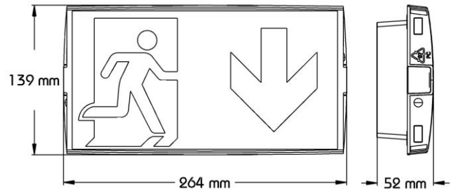
Maßzeichnung
