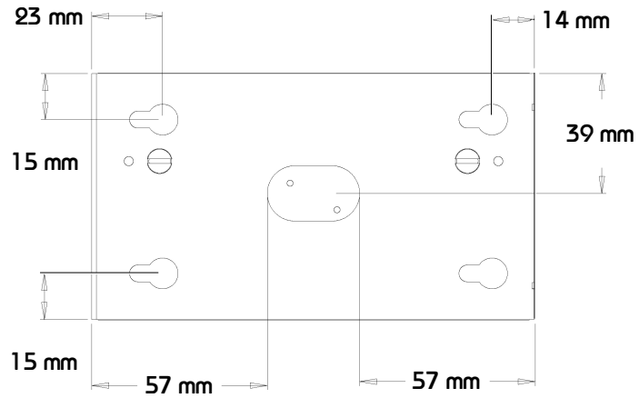
Ansicht Oben
