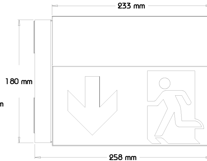
Ansicht Hinten
