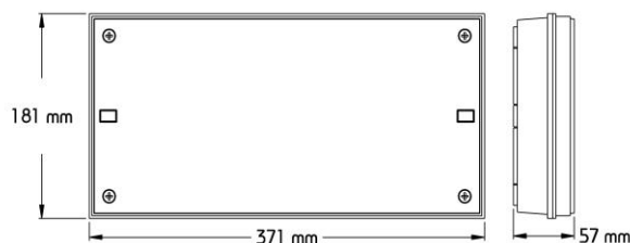
Maßzeichnung
